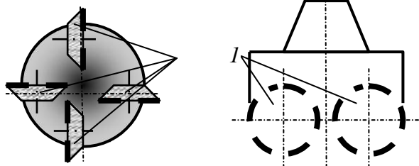
Рис. 1.6. Схема долота с зубчато-дисковыми шарошками
