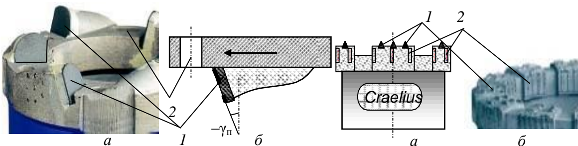
Рис. 1.31. Коронка с поликристаллическими вставками Diapax ( а ) и схема вставки ( б – вид сбоку): 1 – вставка; 2 – отверстия для промывочной жидкости
