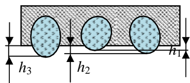
Рис. 1.3. Овализованные алмазы в матрице коронки.
