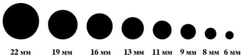
Рис. 2.126. Диаметры резцов долот PDC.
