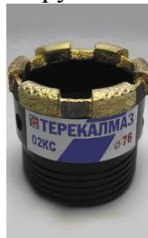
Рис. 2.62. Однослойная буровая коронка 02КС.
